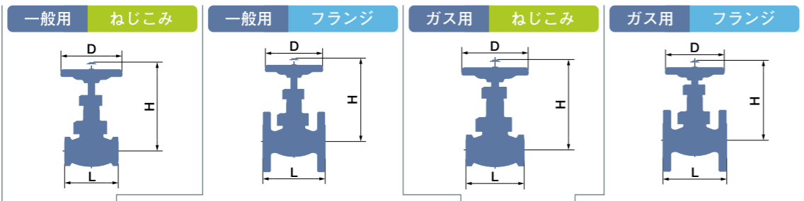
外観図・寸法表 (円)
