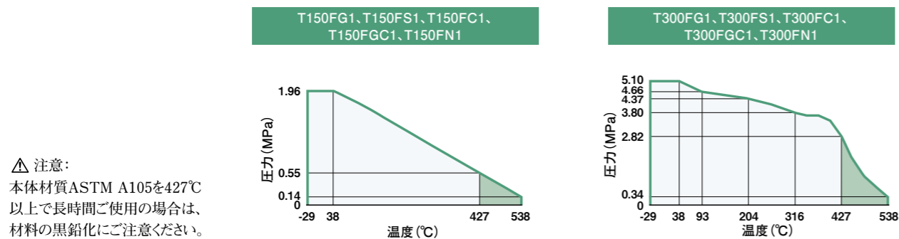
圧力 — 温度レーティング
