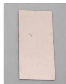
Cu/NVF合金
