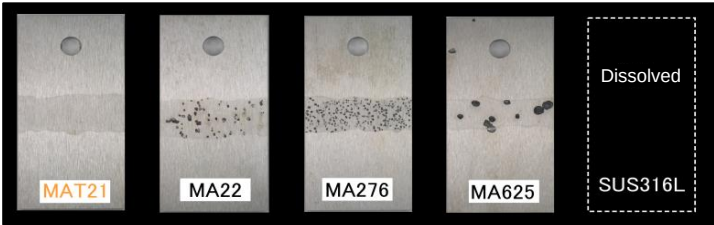
【Pitting Corrosion Test Example】
