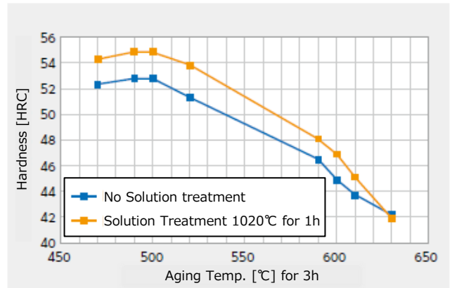
YAG285AMの時効曲線
