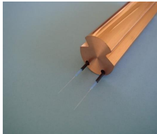
光ファイバを用いた警報機能付きトロリ線
